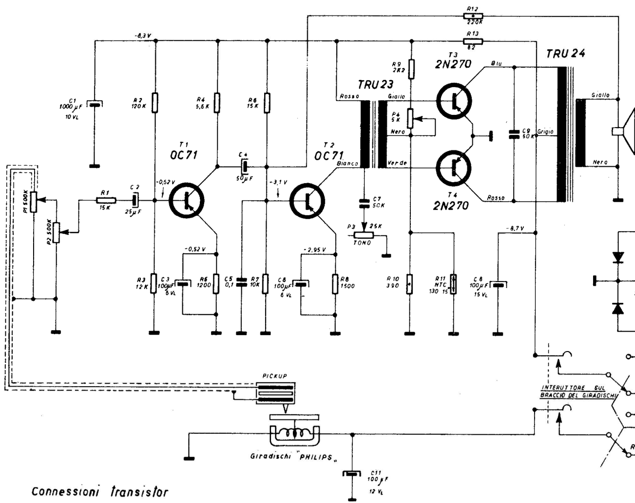
SCHEMA ELETTRICO DELLA FONOVAGLIA A 4 TRANSISTORI Mod. FP 1008 della "VEGA,,
